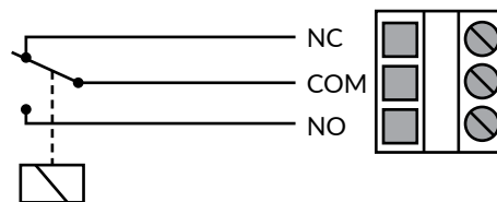
Рисунок 2с - Монтажная электросхема: Реле
