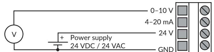
Рисунок 2а - Монтажная электросхема 0-10 V выход
