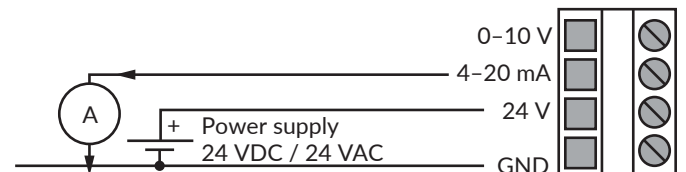
Рисунок 2б - Монтажная электросхема 4-20 mA выход
