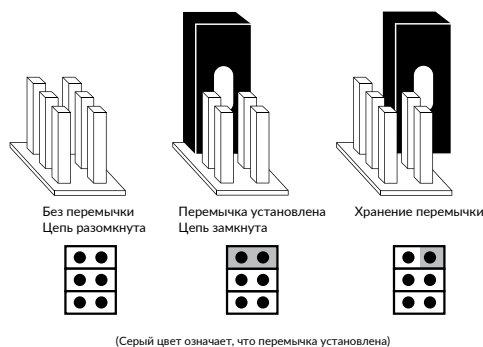
Рисунок 3 - Установка перемычки
